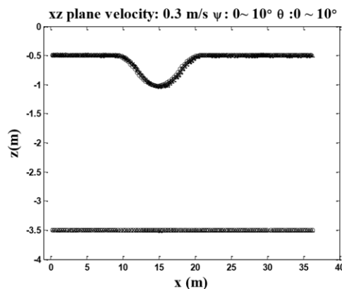
(d) UKF-SLAM sequential
